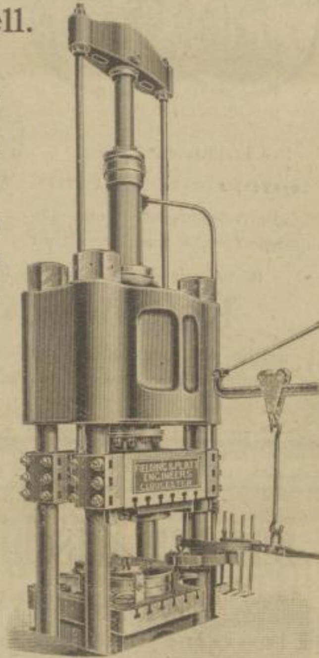
Schmiedepresse für Waggonräder.
