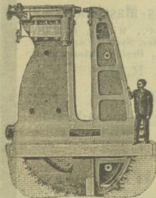
Patent. hydraul. stationäre Nietmaschine von 3250 mm Ausstattung, 150 To. Druck.
