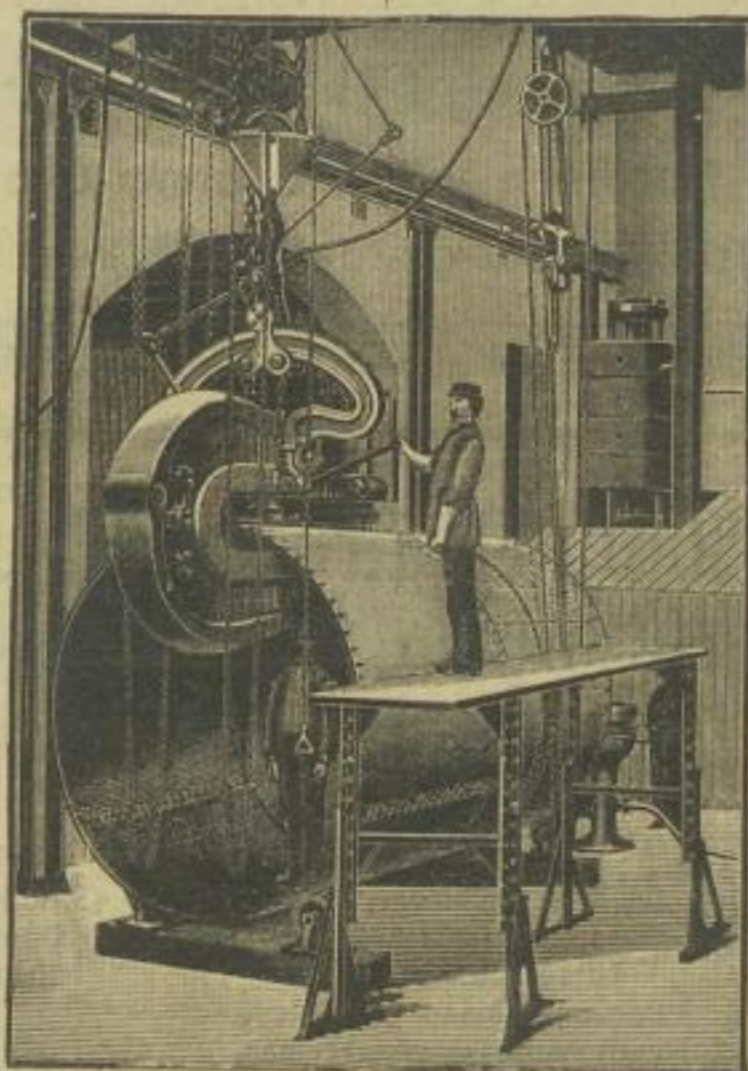
Hydraulische Nietanlage.
