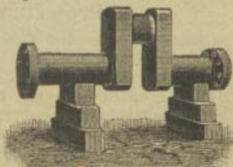
Schiffskurbelachse. 2520
