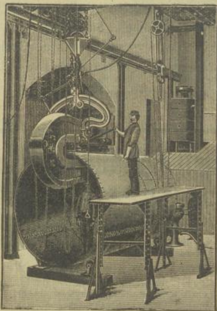
Hydraulische Nietanlage.
