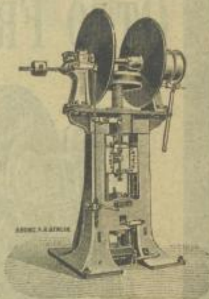
Frictionspresse für Schrauben, Nieten, Schienennägel u. s. w.
