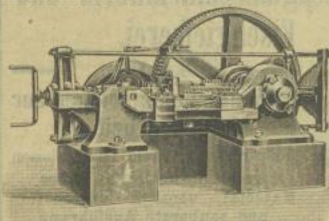
Mutterpresse.
