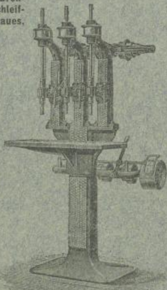
Ein- bis vierspindlige Schnellbohrmaschine, Serie G. mit Gefühlshebel. 3006e
