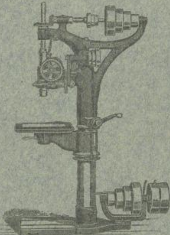
Freist. Säulenbohrmaschine, Modell CB. mit feststehend. Spindelkopf, selbsthät. Nieder-gang der Bohrspindel u. selbsthät. Ausschaltung.
