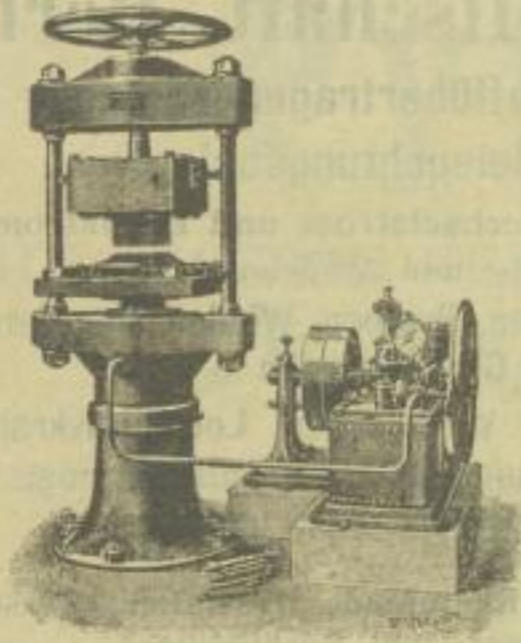
Hydraul. Presse H. P. 50.
