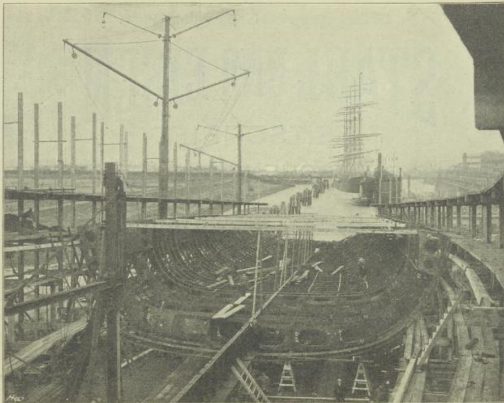
FIGUR 1. LINIENSCHIFF „KAISER KARL DER GROSSE“. Baustadium am 1. Januar 1899.
