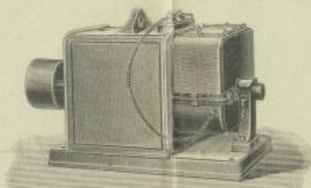
Fig. 1. Geschlossener Motor Modell PA.
