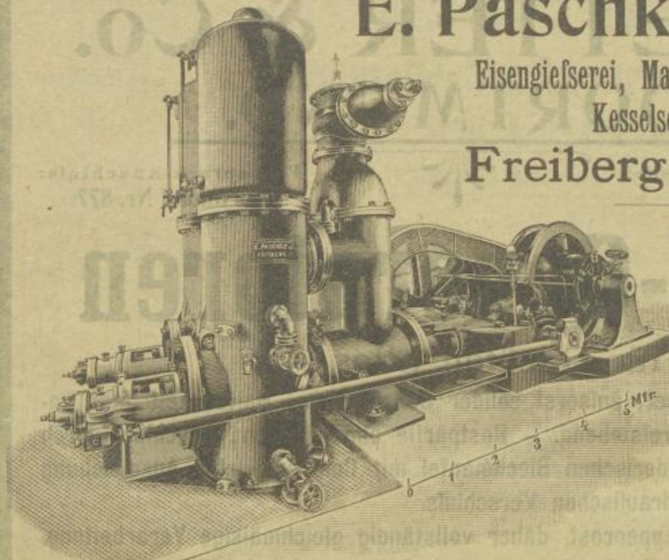
5056 Elektrisch betriebene Zwillings-Differentialplungerpumpe von 13 cbm minuti. Leistung.
