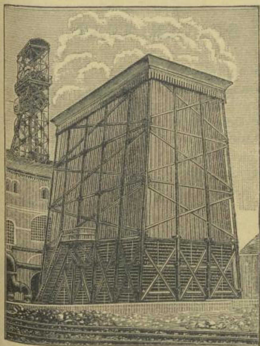
Kaminkühler für 750 cbm Wasser pro Stunde.
