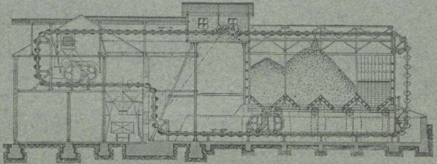
Conveyoranlage, ausgeführt für die Königl. Berginspektion Dudweiler.
