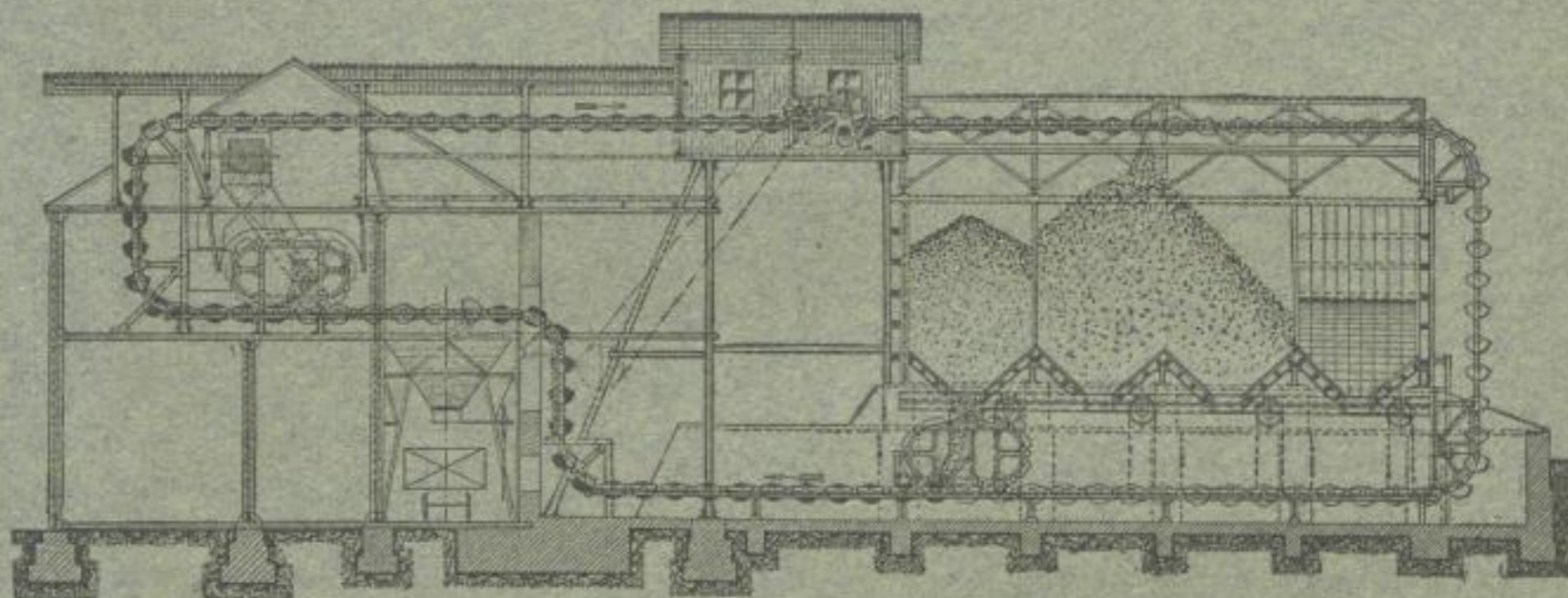
Conveyoranlage, ausgeführt für die Königl. Berginspektion Dudweiler.
