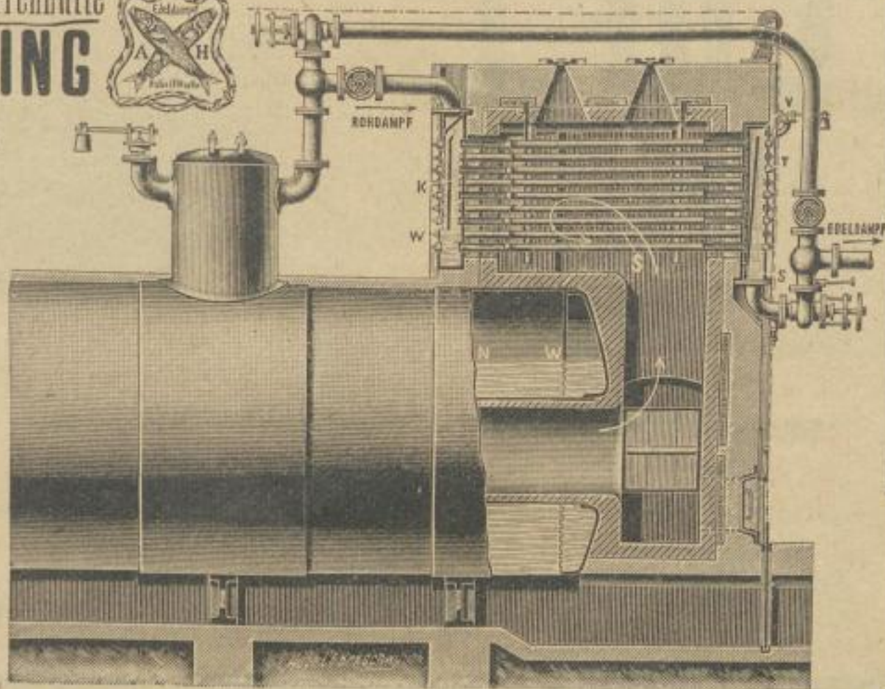
Rauchgasausnützer (Engröhrige Economiser).
