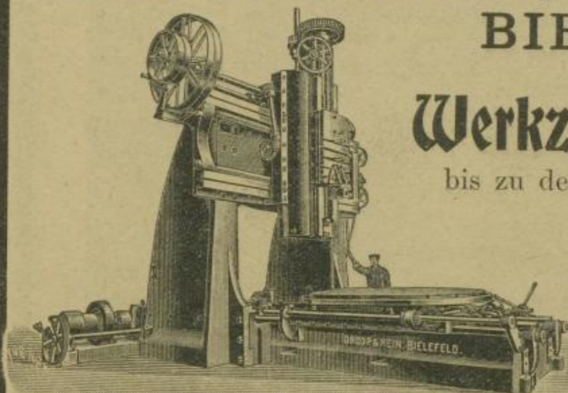
Vertikale Hobelmaschine von 2500 mm Werkzeughub.
