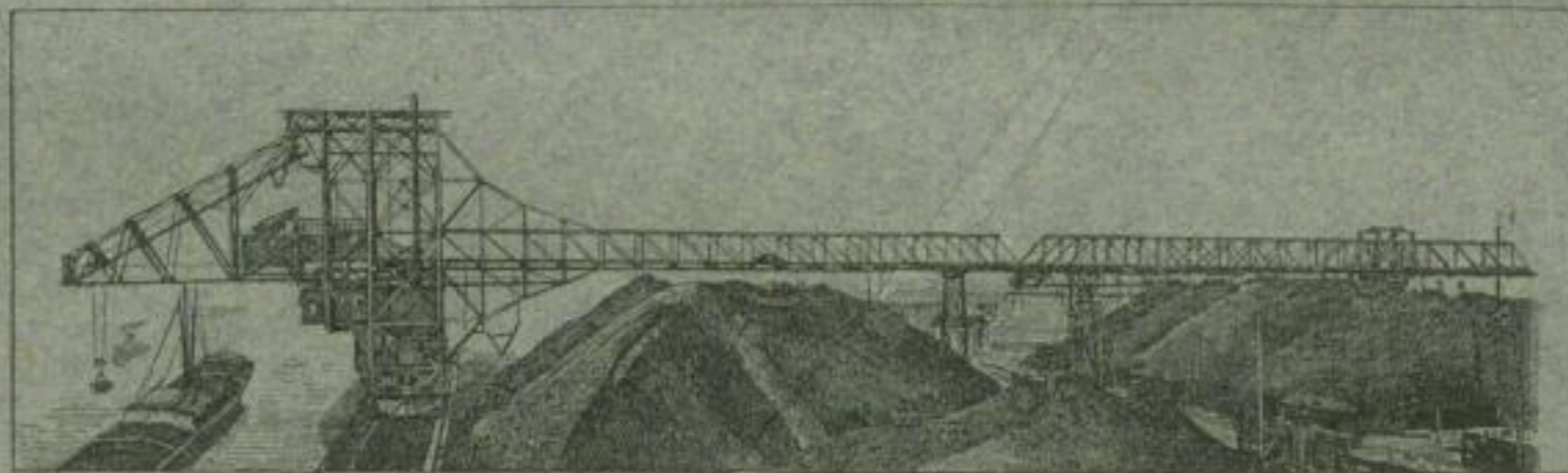
2 Elevatoren in Verbindung mit automatischen Bahnen, ausgeführt für den Schalker Gruben- und Hüttenverein, Abth. Duisburg.
