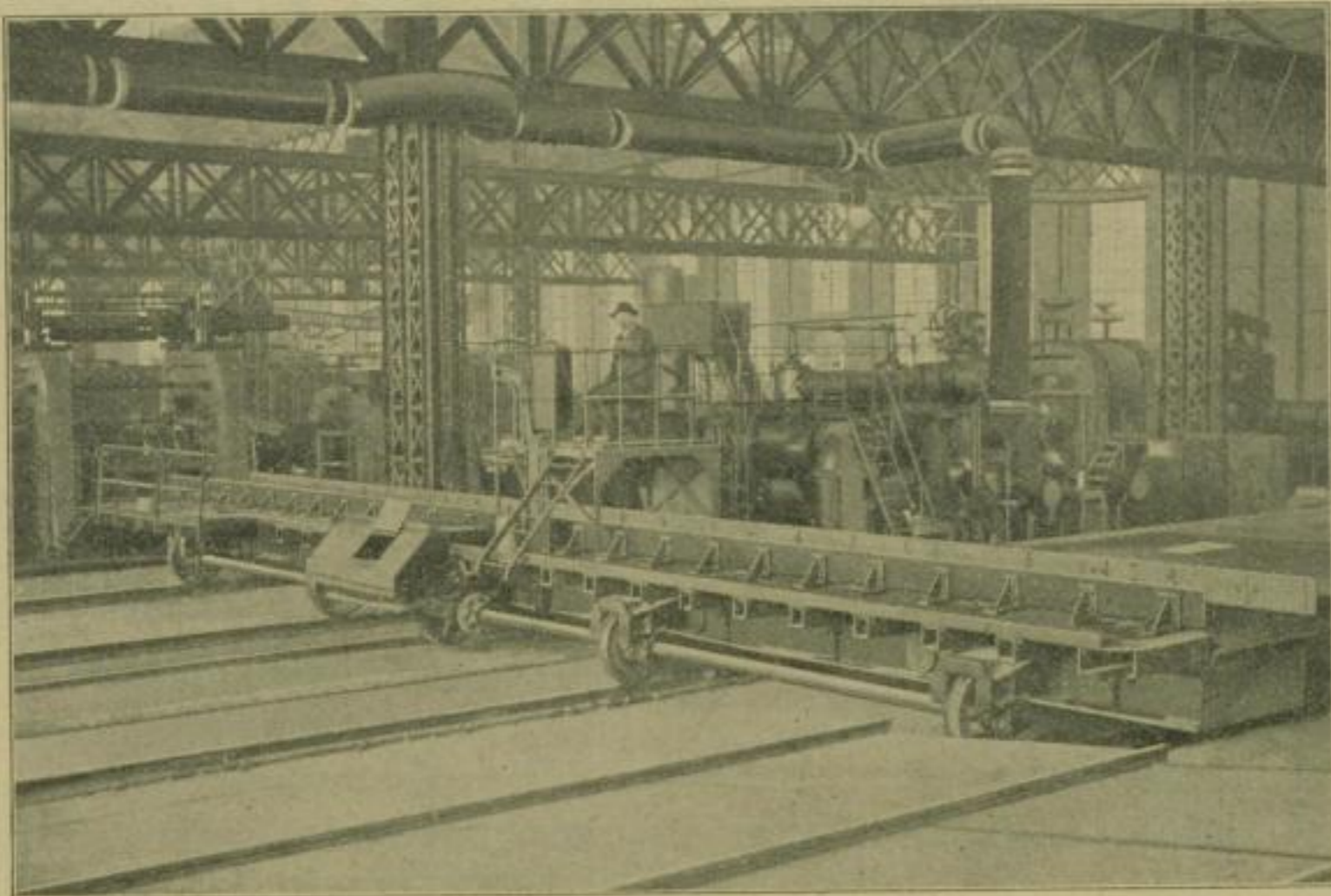
850er Träger-Duo mit elektr. angetriebenen fahrbaren Rollgängen, geliefert an Friedenshütte und Société Dniéprovienné.
