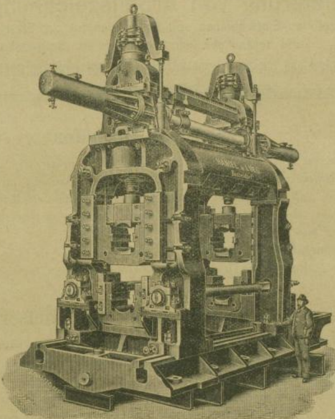
Blockwalzgerüst.
