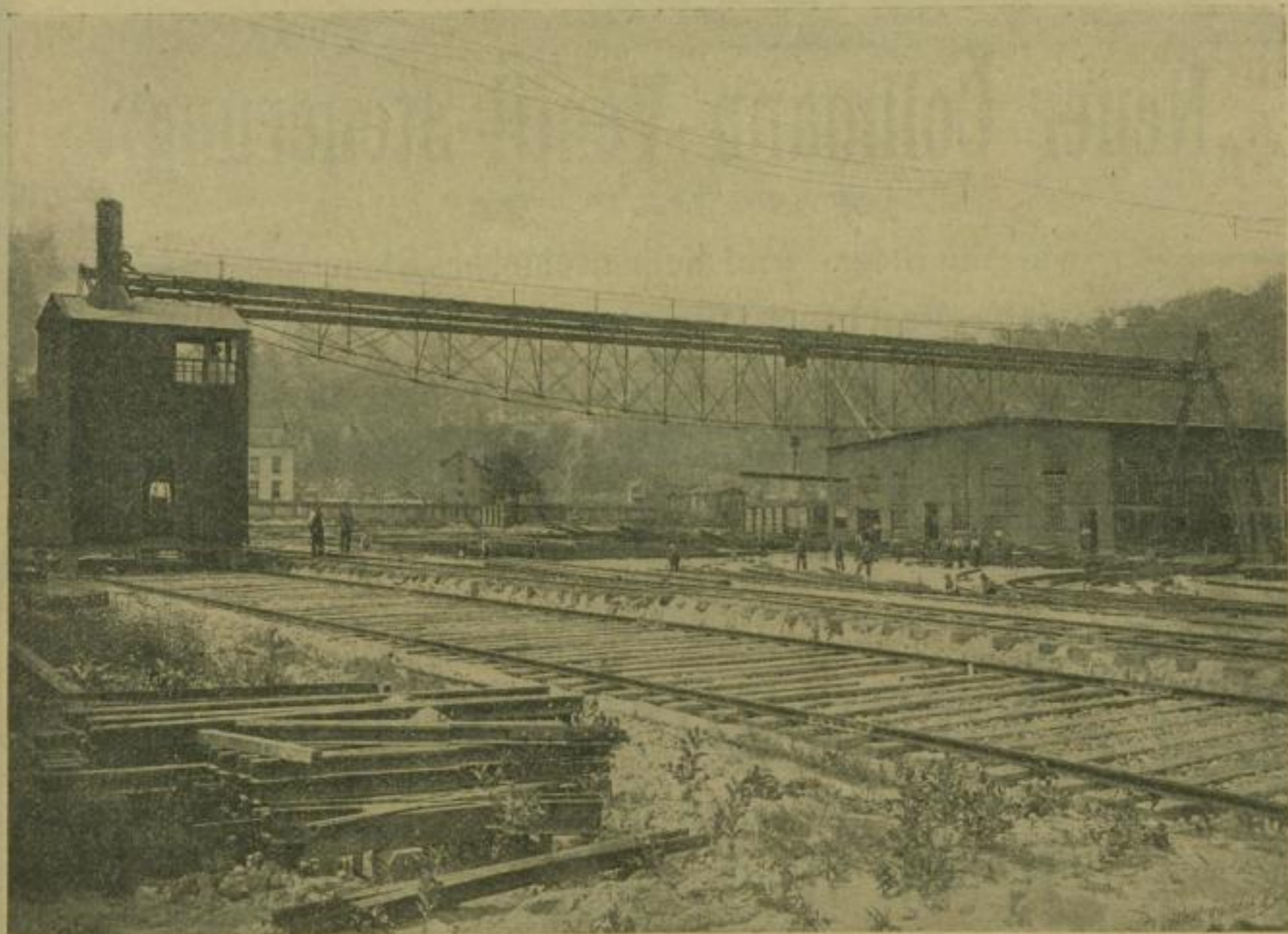
5 Tonnen-Brückenlaufkran von 190 Fuß Spannweite der Lorain-Steel Co., Johnstown, Pa.
