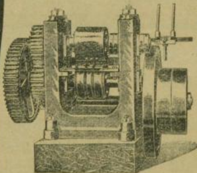
Walzmaschine zum Absetzen, Profilieren u. s. w. von Eisenstäben.
