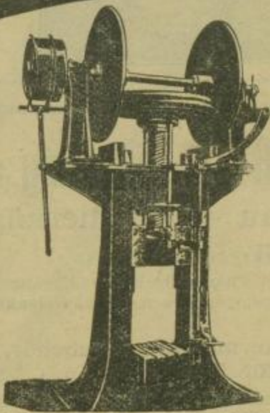
Frictionspresse für Gesenkschmiedearbeit
