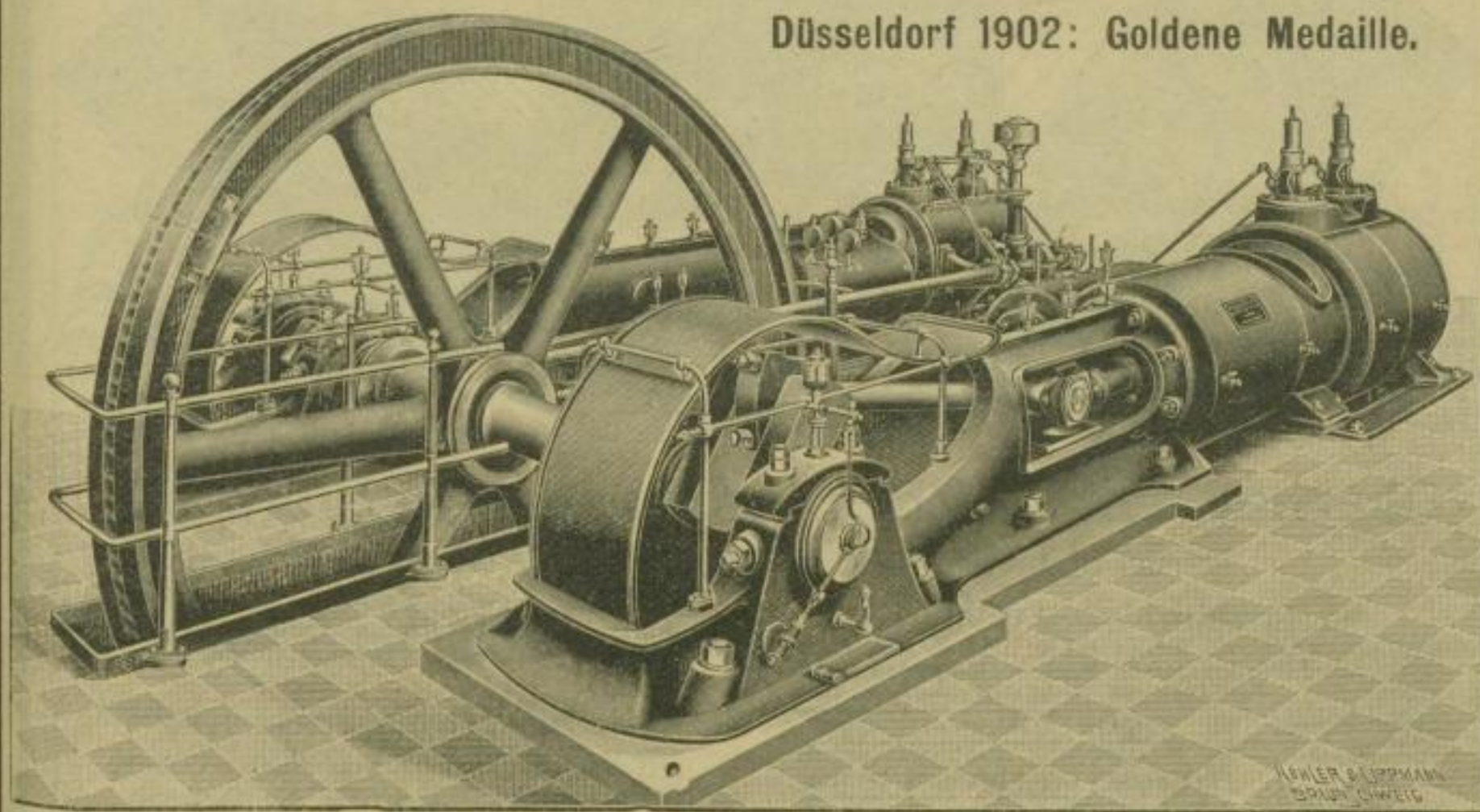
2686a Mit Dampfmaschine gekuppelter Verbund-Kompressor. 7000 cbm Stundeleistung auf 6 Atm.
