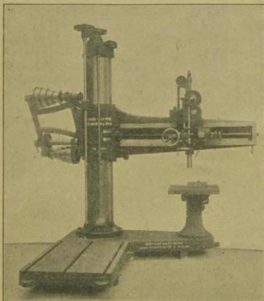
Halbuniversal-Radialbohrmaschine.
