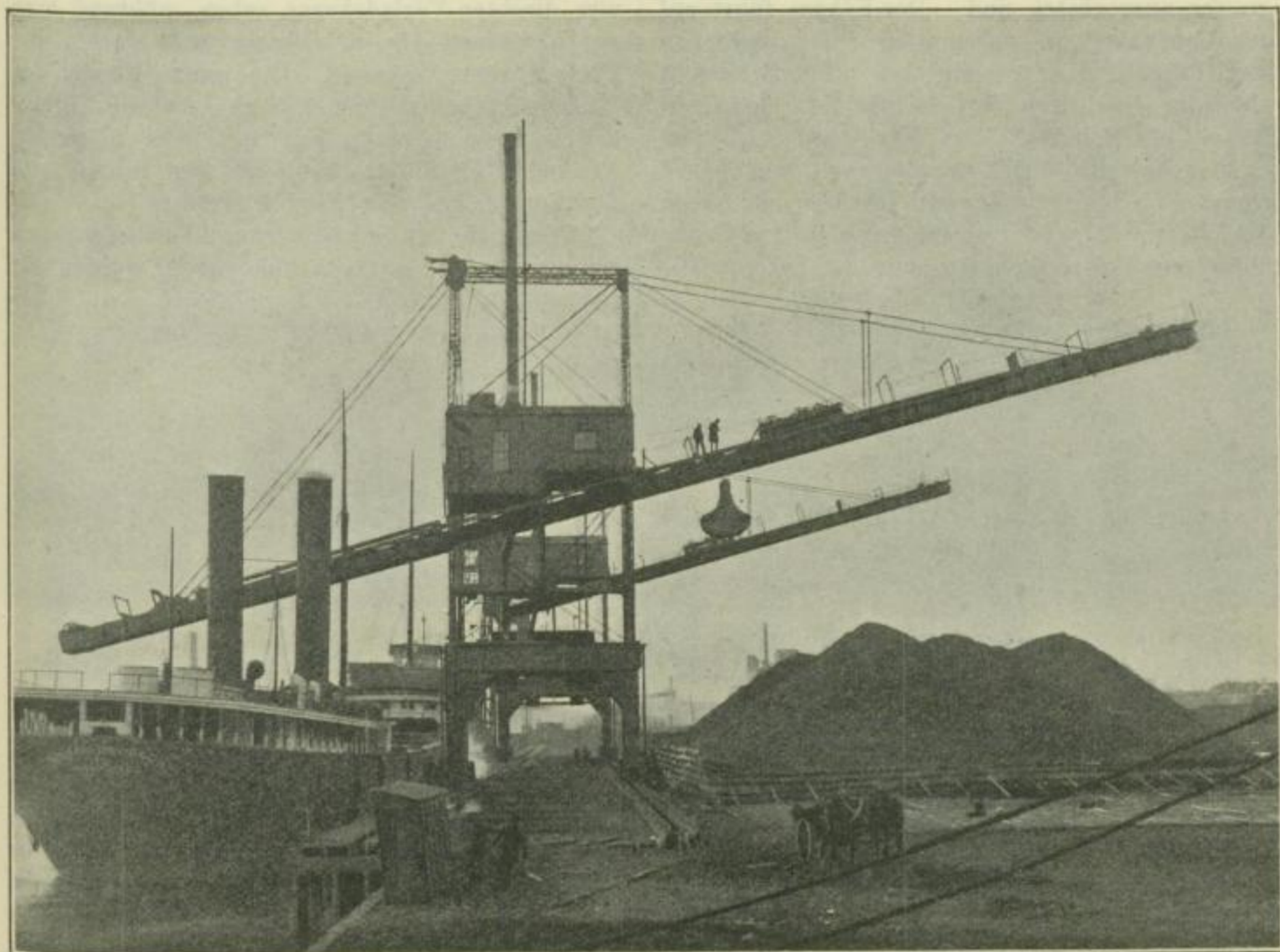
Abbildung 11. Direkte Verladekrane für die Solvay Process Co., Milwaukee, Wisc.
