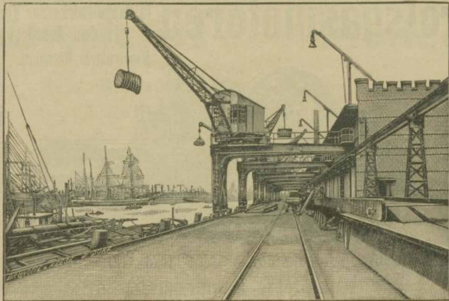
Elektr. Hafen-Kran (Halbportalkran) 3 t Tragkr., 11 m Ausladung.
