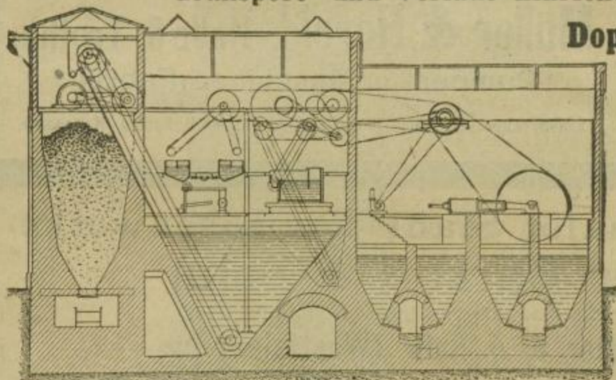
Kokskohlen - Wäsche.
