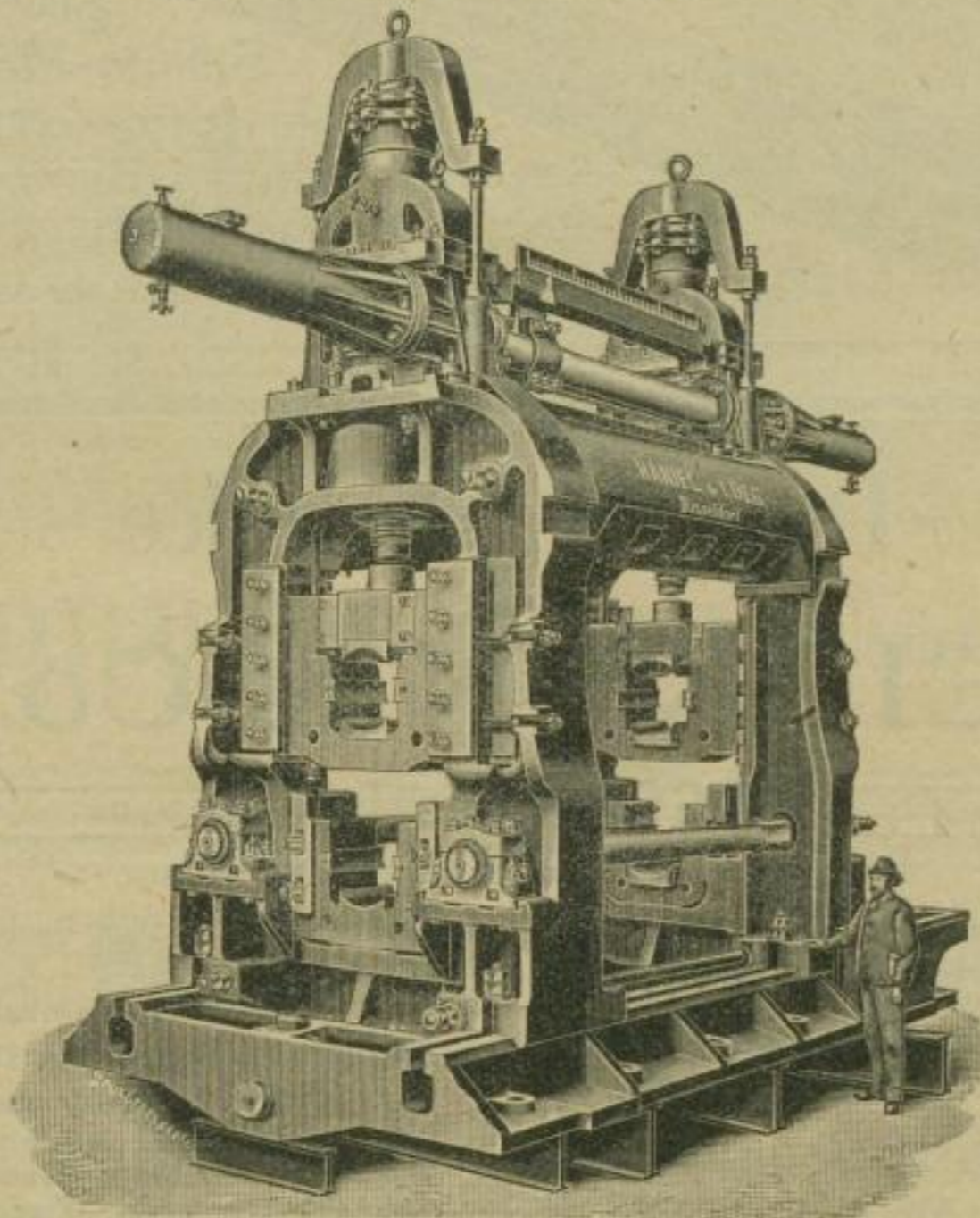
Blockwalzgerüst.
