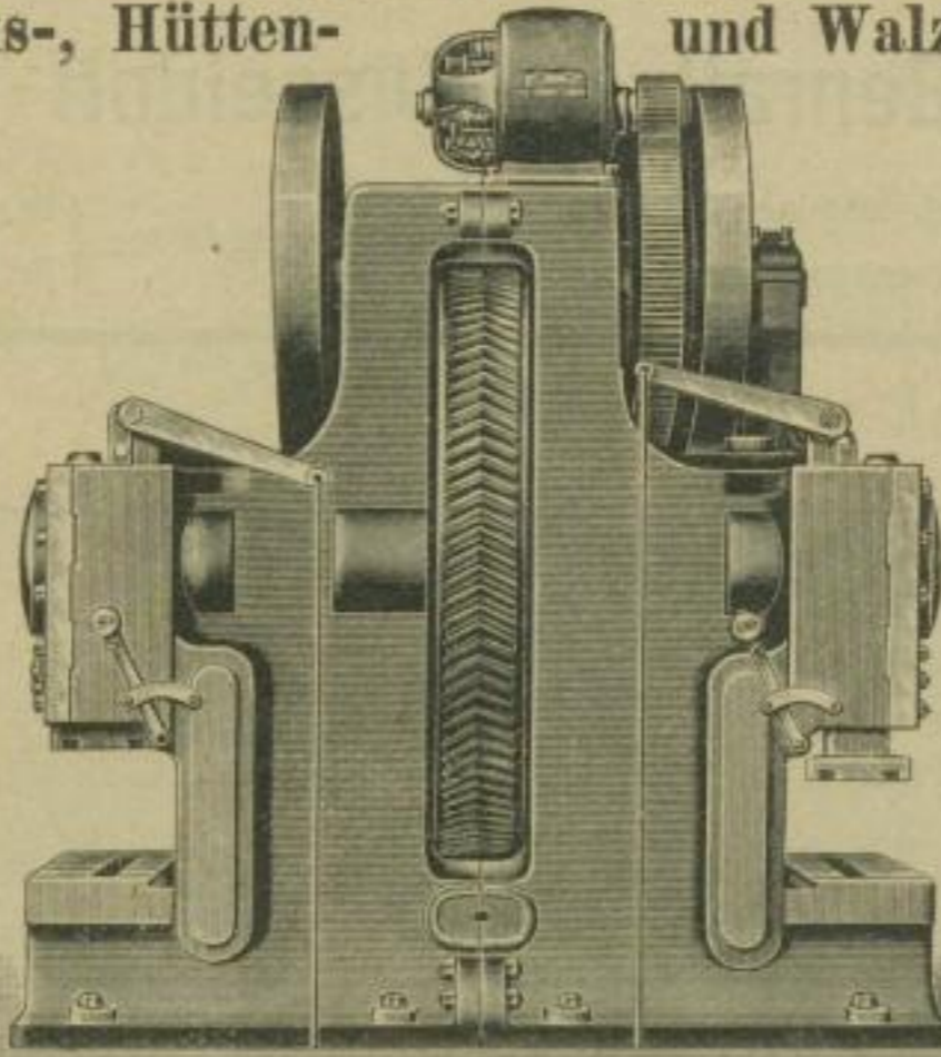
Doppelstanze für 500 000 Ko. Druck.
