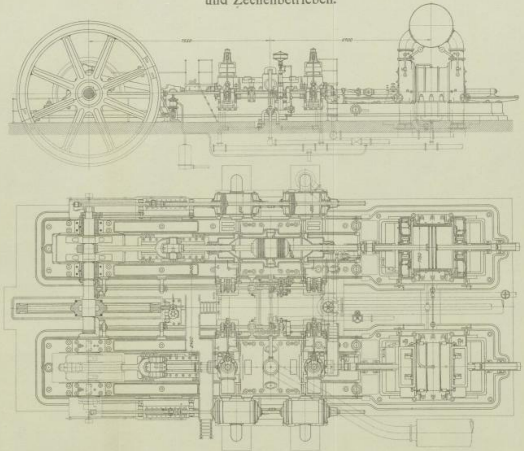
Zwillings-Hochofengas-Gebläsemaschine der Maschinenbau-Aktien-Gesellschaft vorm. Gebr. Klein in Dahlbruch.
