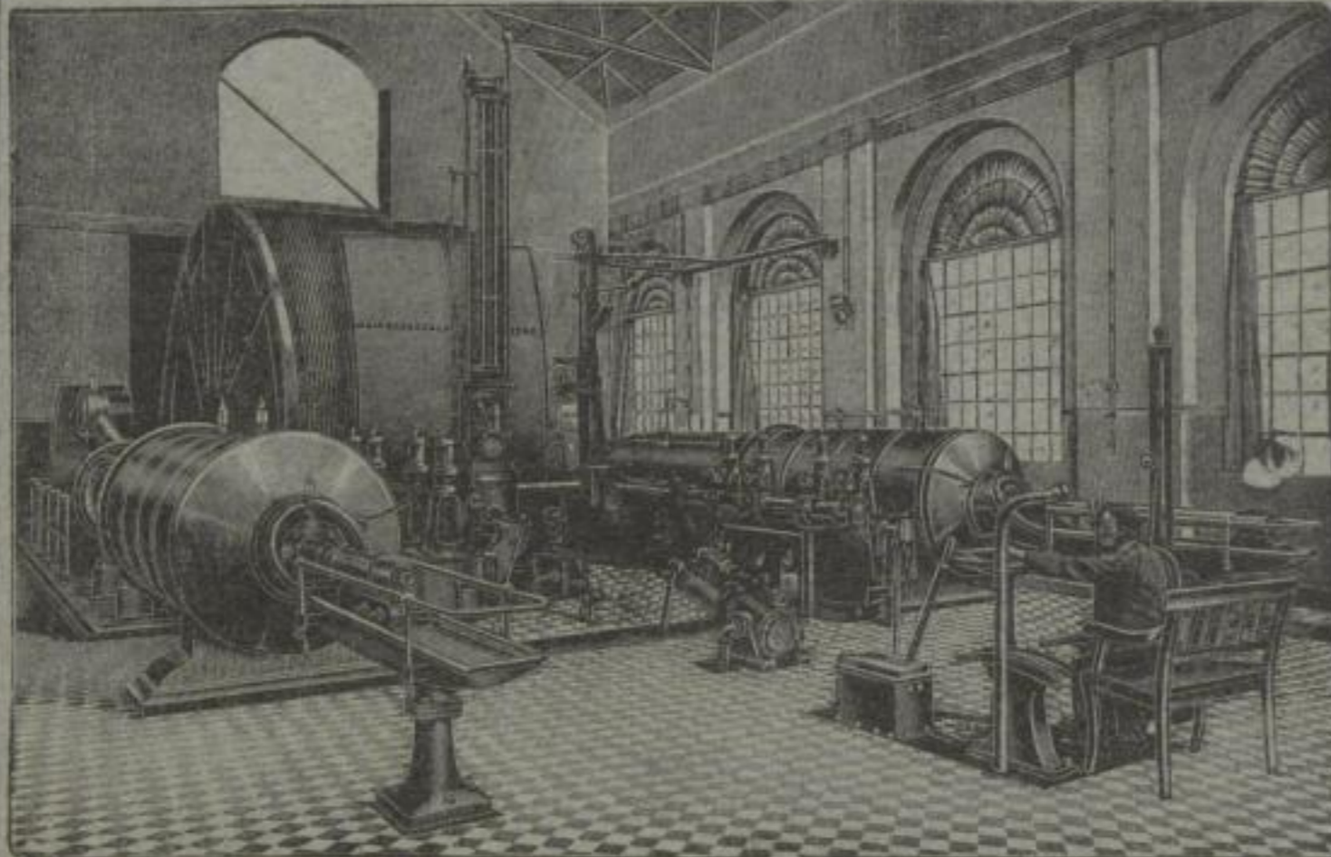
Zwillings-Fördermaschine für eine Leistung von 150 t in der Stunde bei 600 m Cente, aufgestellt auf der Kruppischen Zeche Hannibal.
