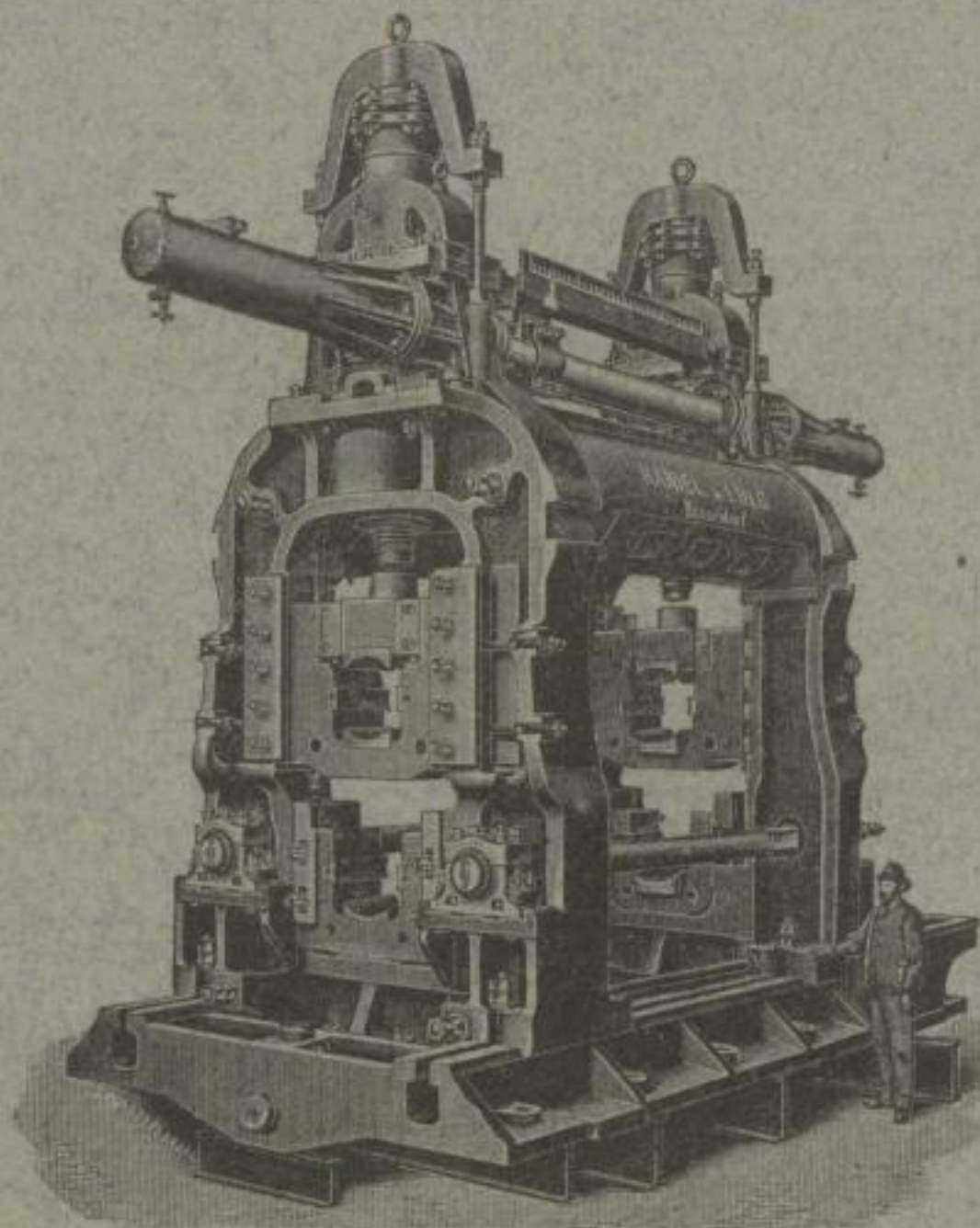
Blockwalzgerüst.
