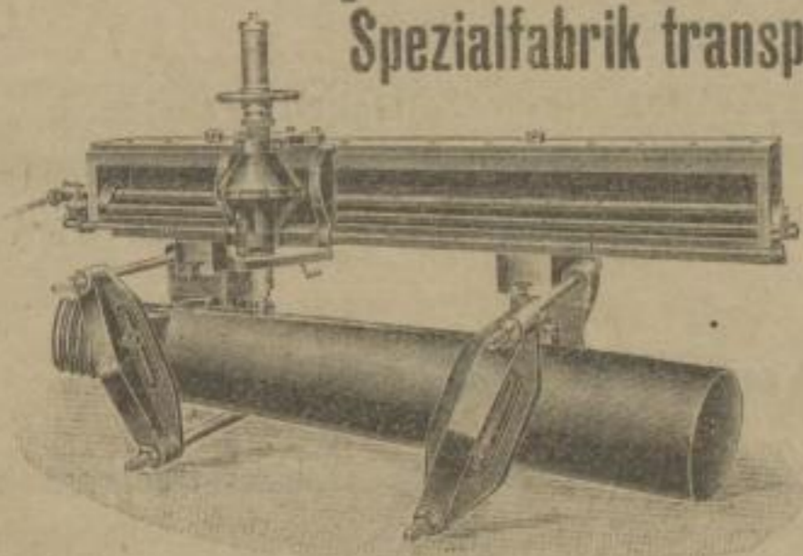
Nutenfräs-Maschine für zyl. u. kon. Wellen bis 800 mm Dmr.
