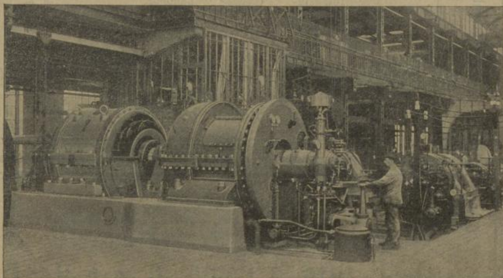
3000 KW.-Turbine im Prüffeld der Turbinenfabrik.
