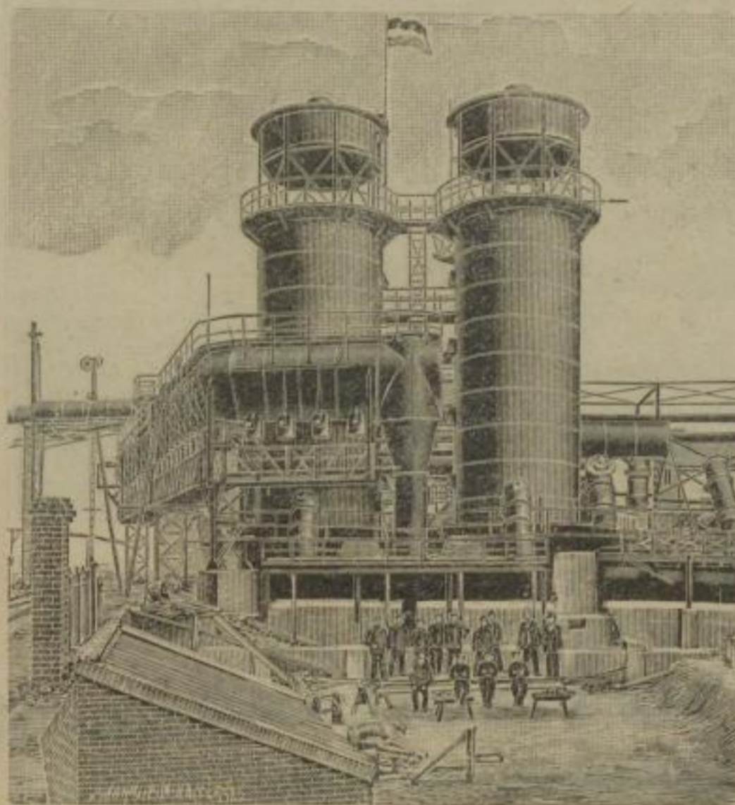
Gicht-Gas-Reinigungs-Anlage, ausgeführt für ein Hüttenwerk in Westfalen.
