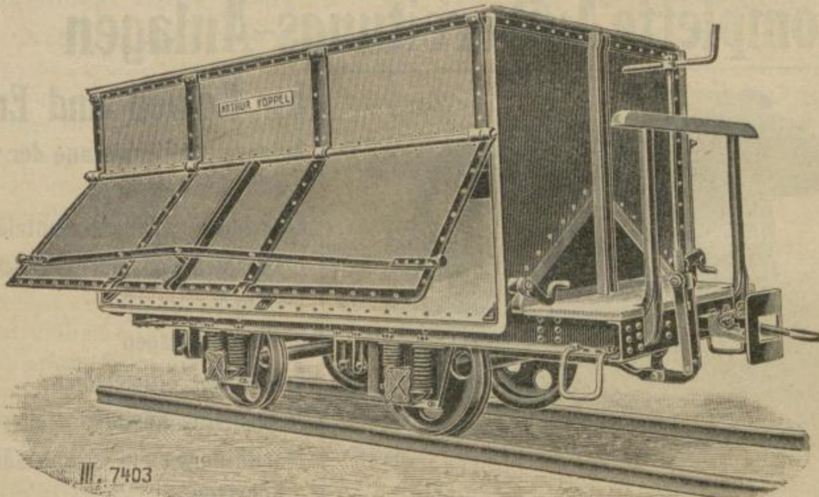
Sattelwagen für Lokomotivbetrieb.
