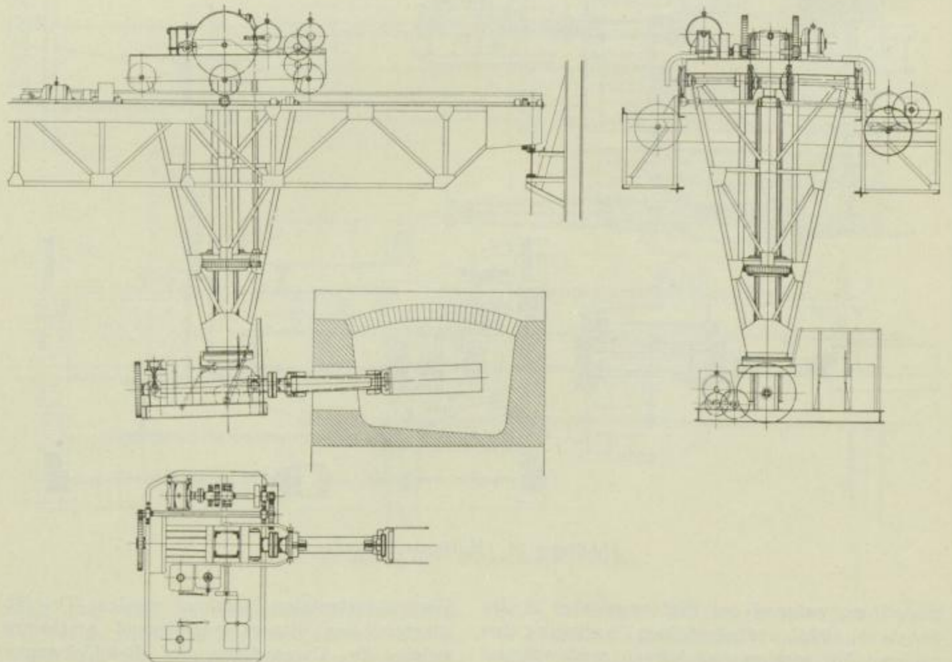
Abbildung 36. Muldenbeschickkran mit schrägsteher Säule.
