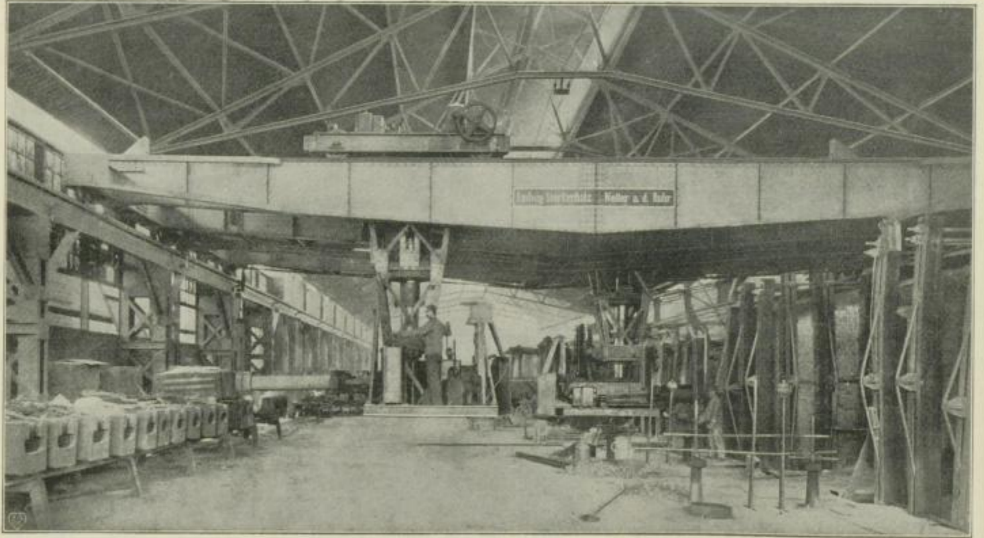
Abbildung 35. Ansicht des Muldenbeschickkrans auf Abbildung 34.
