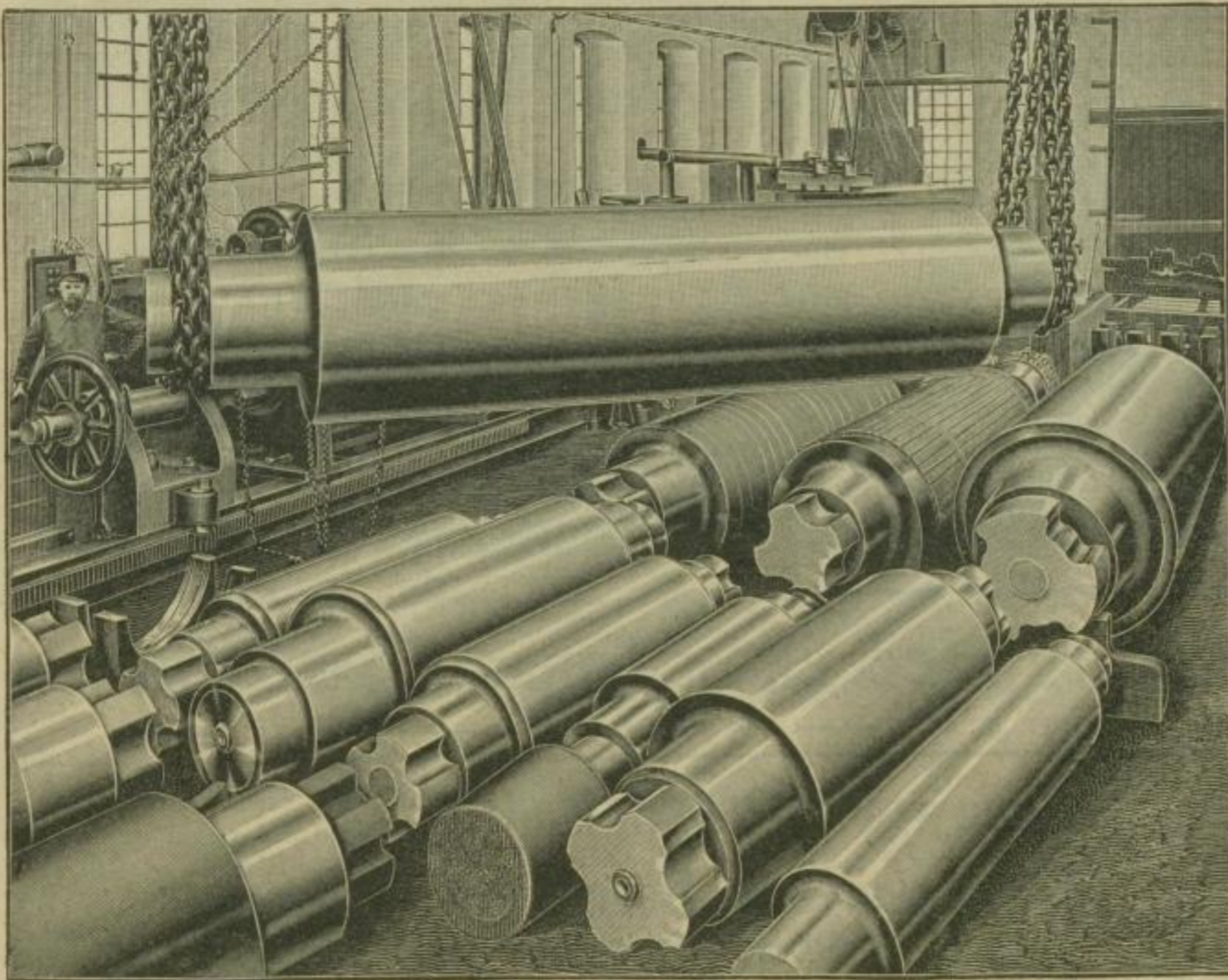
Gruppe von Blech-Hartwalzen nach „Patent Peipers“.
