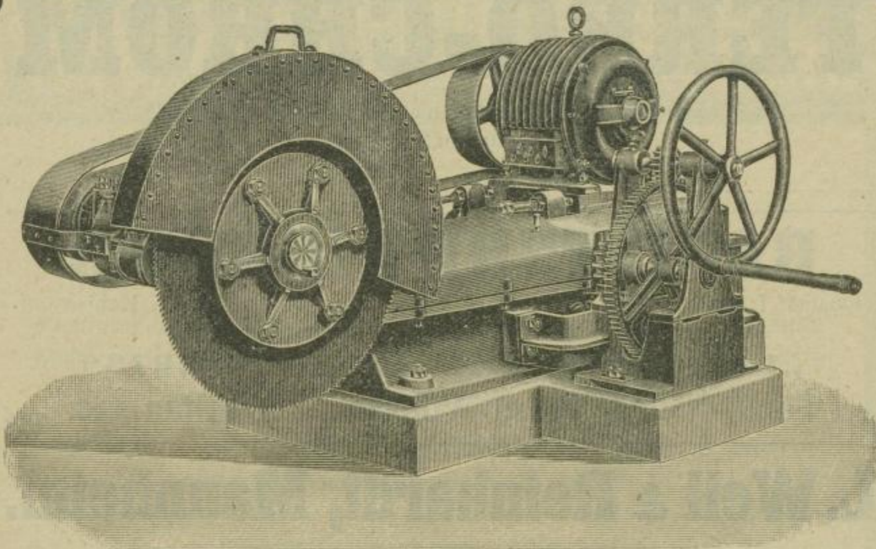
Schlittensäge für Knüppel, Stabeisen und kleinere Träger.
