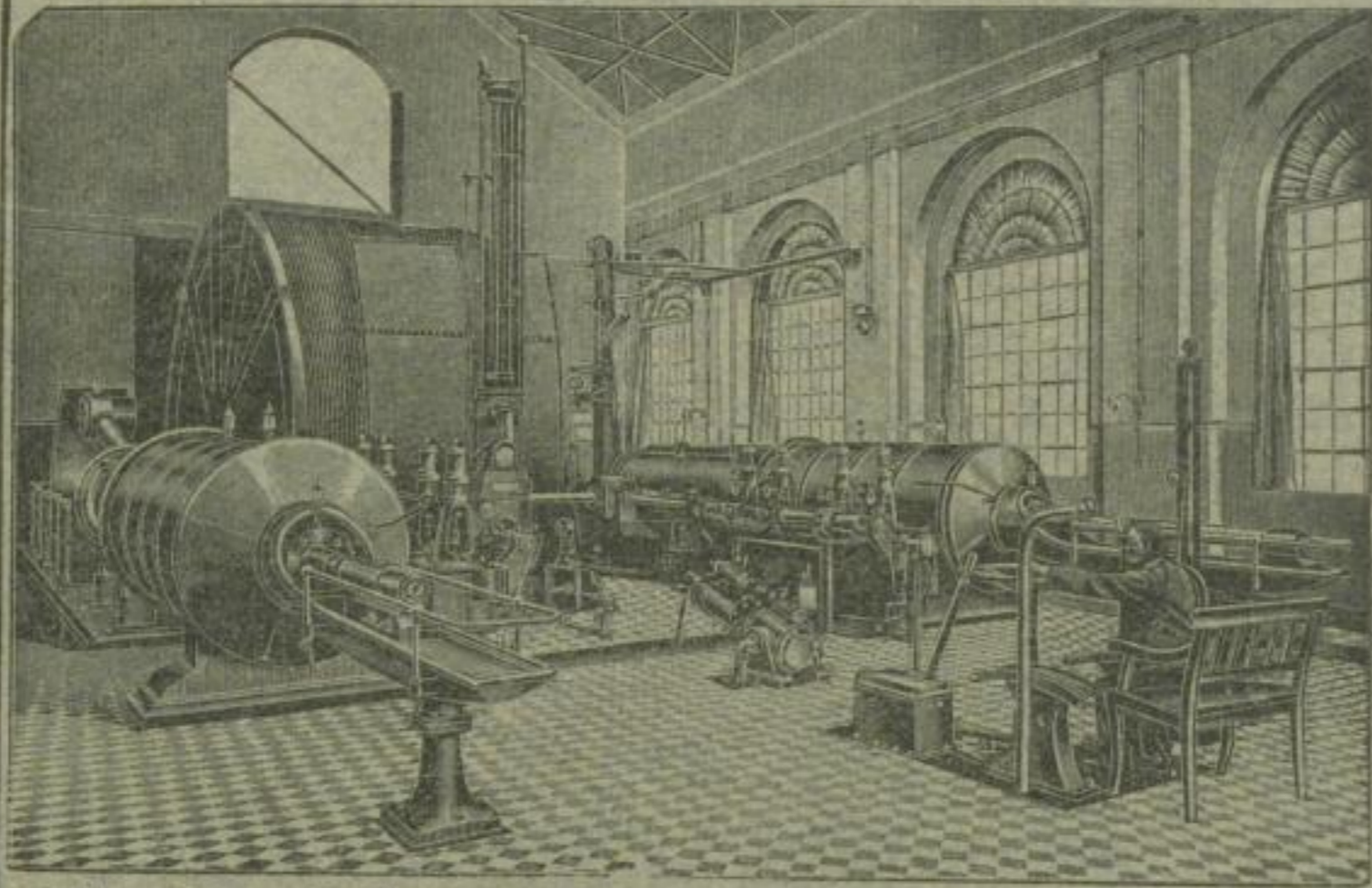
Zwillings-Fördermaschine für eine Leistung von 150 t in der Stunde bei 600 m Cente, aufgestellt auf der Kruppschen Zeche Hannibal.
