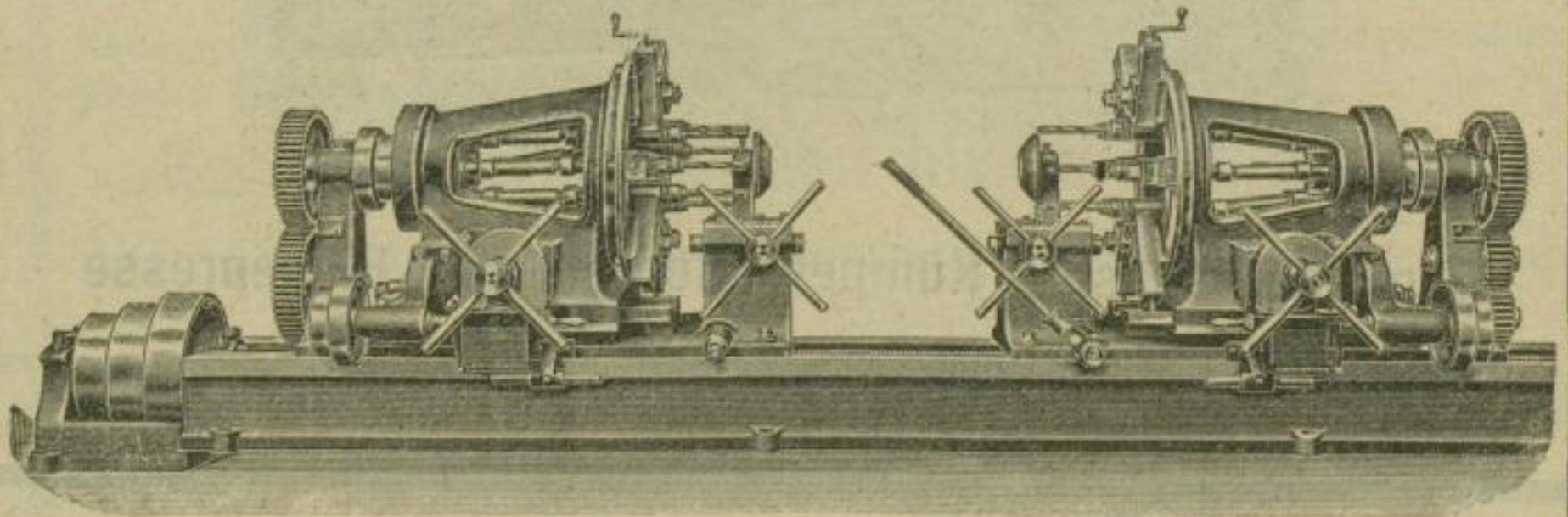
Doppelte sechsspindelige Flanschenbohrmaschine.
