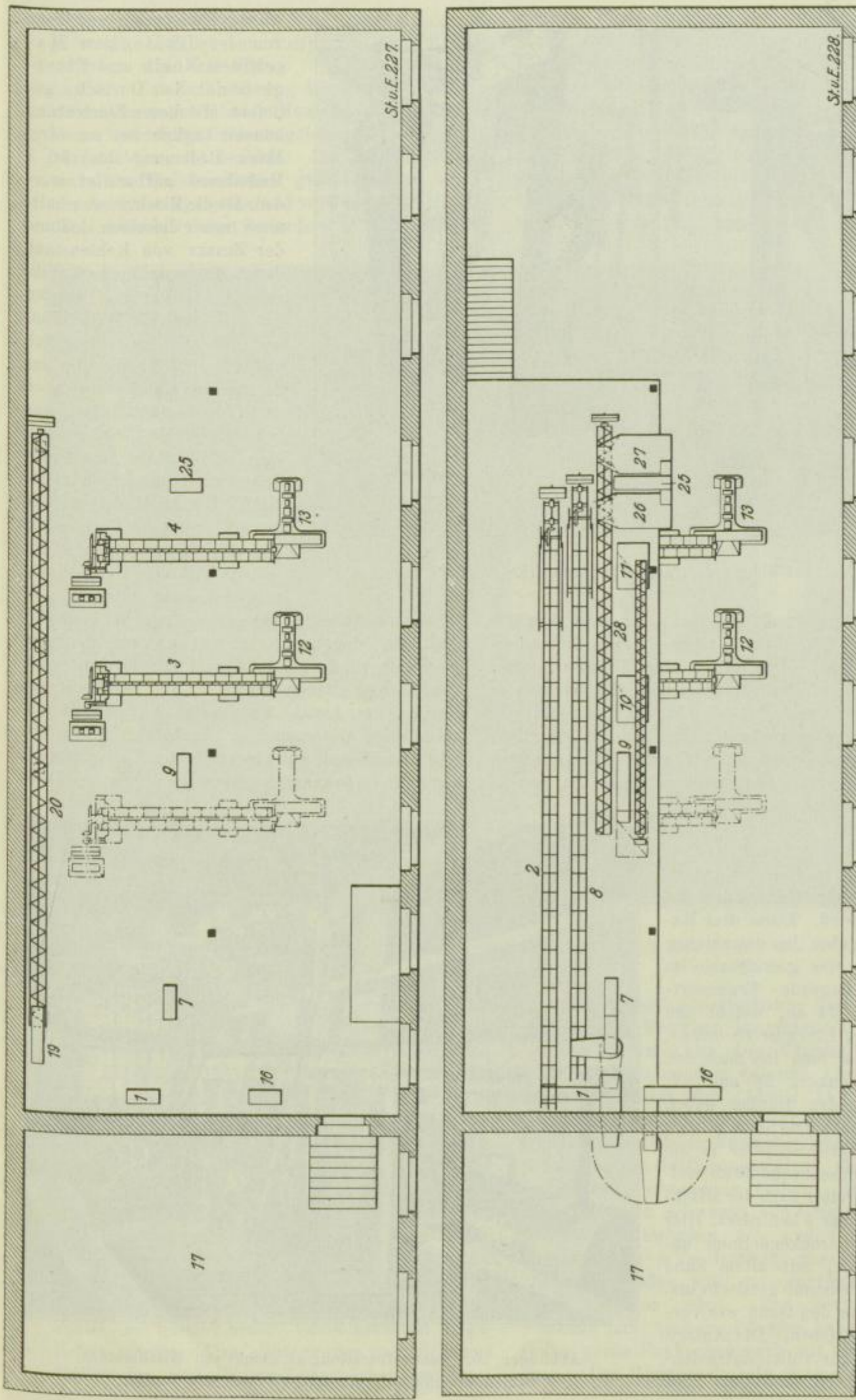
Abbildung 6 bis 8. Sandaufbereitung.
