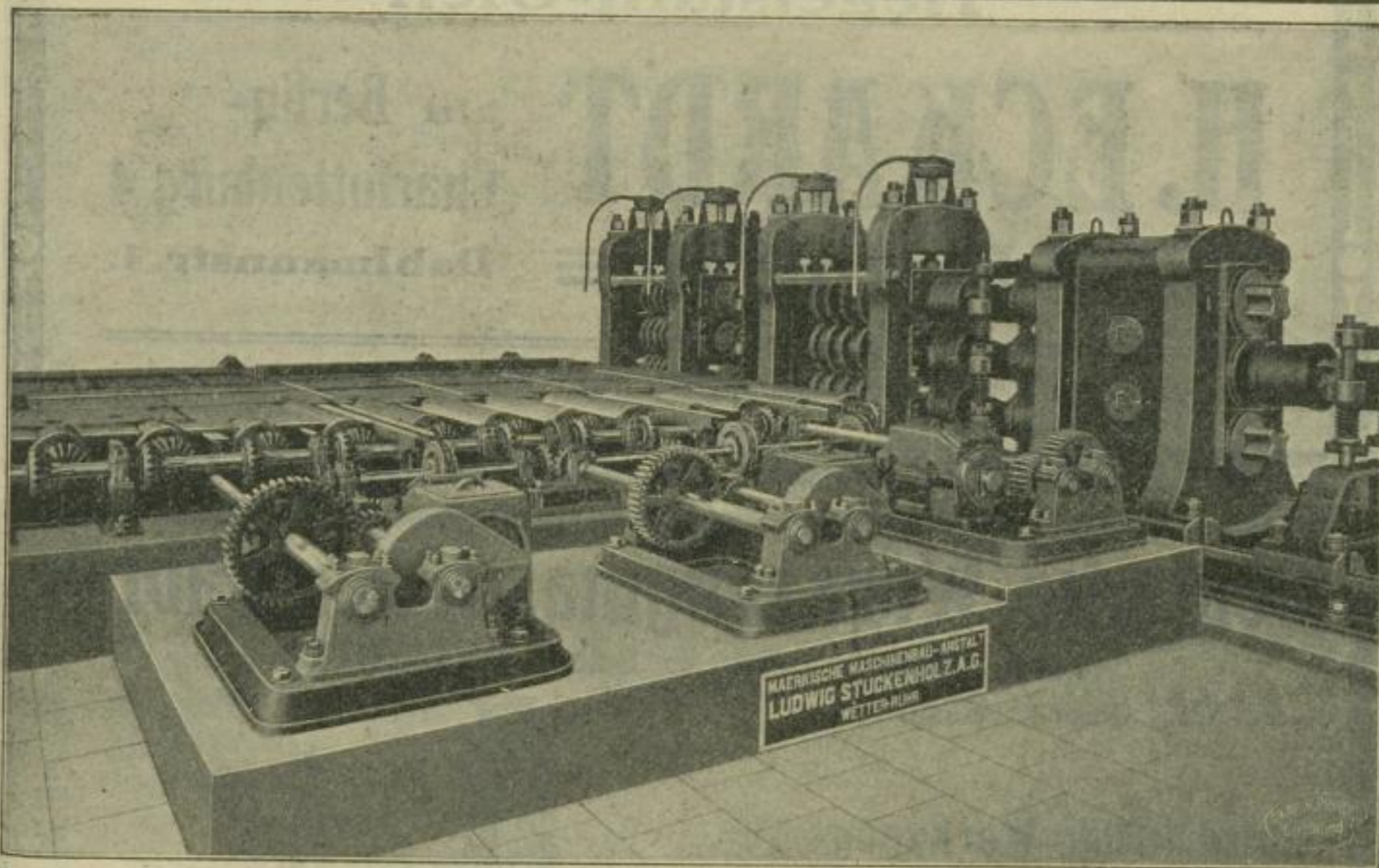
Triowalzwerk für Stabeisen.
