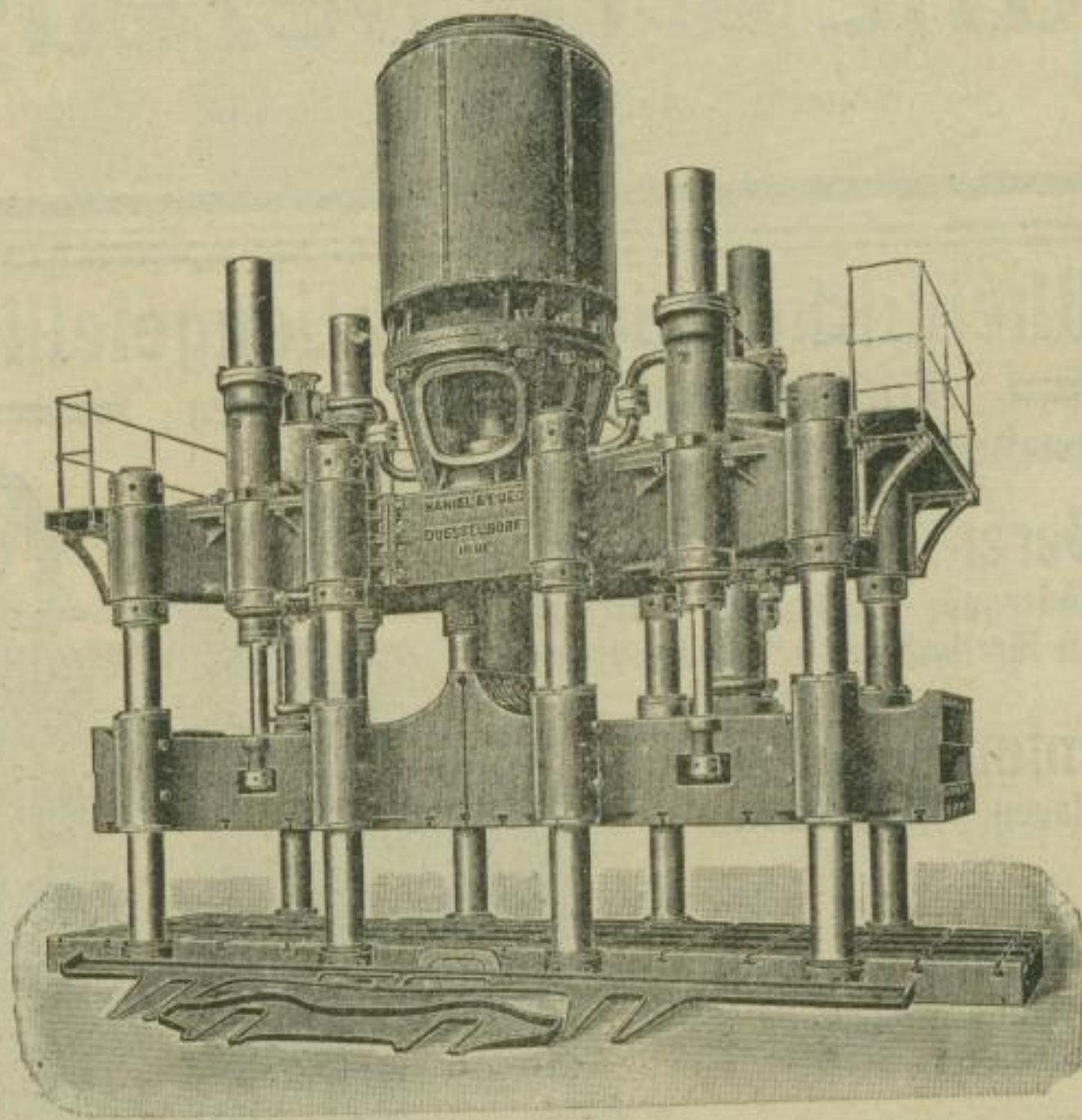
Dampfhydraulische Kumpel-, Bördel- und Biegepresse für Stücke bis zu 12 m Länge.
