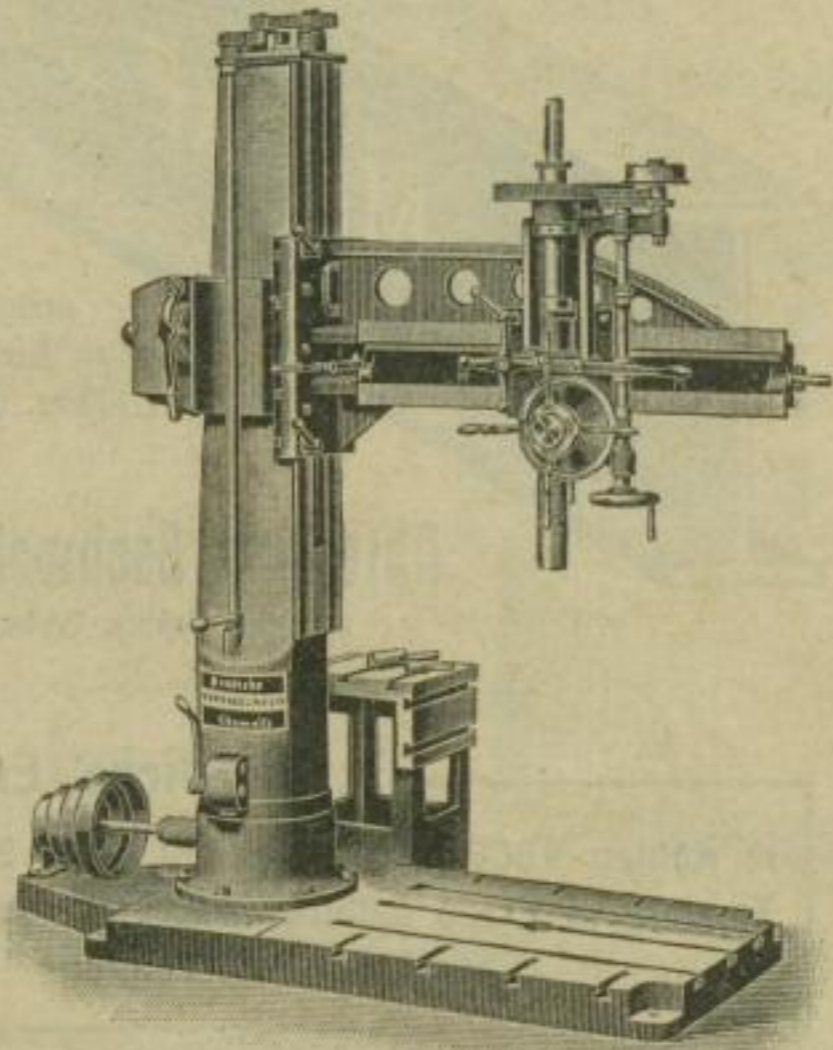
Freistehende Radial-Bohrmaschine.
