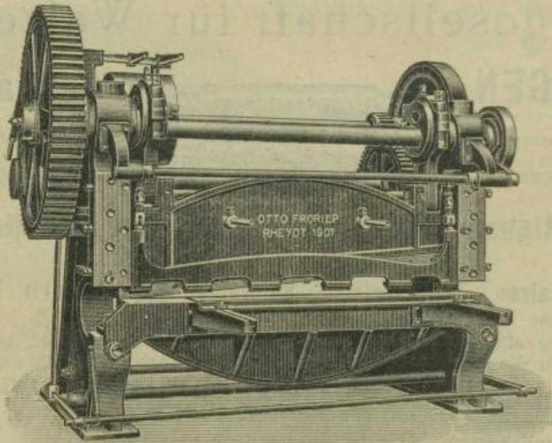
Kurbelschere mit Niederhalter für Bleche bis 10 mm stark, 2000 mm breit.
