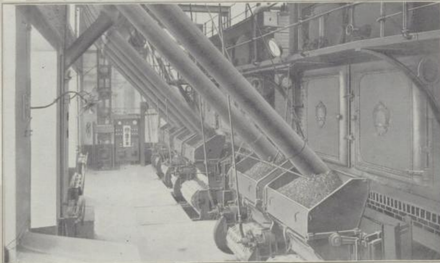
Laederich & Co., Akt.-Ges., Spinnereien und Webereien, Mülhausen i. Els. Drei Babcock & Wilcox Patent-Wasserrohr-Dampfkessel von je 325 qm Heizfläche, mit Überhitzern und Kettenrosten.
