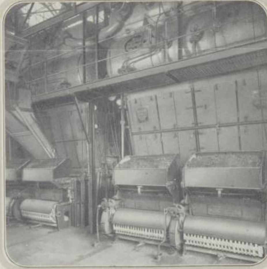
Allgemeine Elektrizitäts-Gesellschaft, Abt. Turbinenfabrik, Berlin NW. ■ Drei Babcock & Wilcox-Hochleistungskessel von je 268 qm Heizfläche, mit Überhitzern und Kettenrosten.
