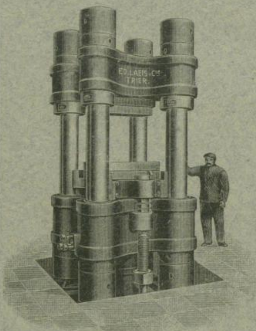
Hydr. Flanschenpresse für 1600 000 kg Preßdruck bei 400 Atm. Wasserdruck.
