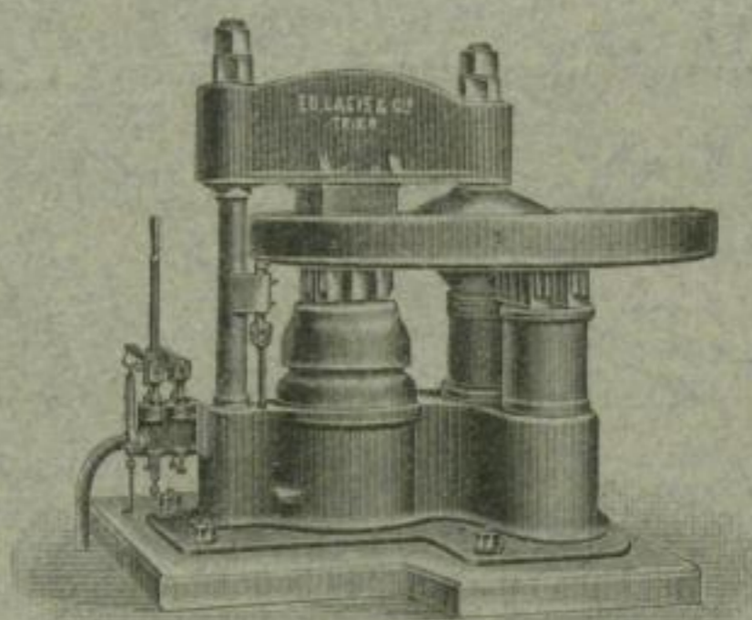
Hydr. Presse mit Drehtisch zur Fabrikat. von Dinas-, Silica- u. Schamottesteinen.
