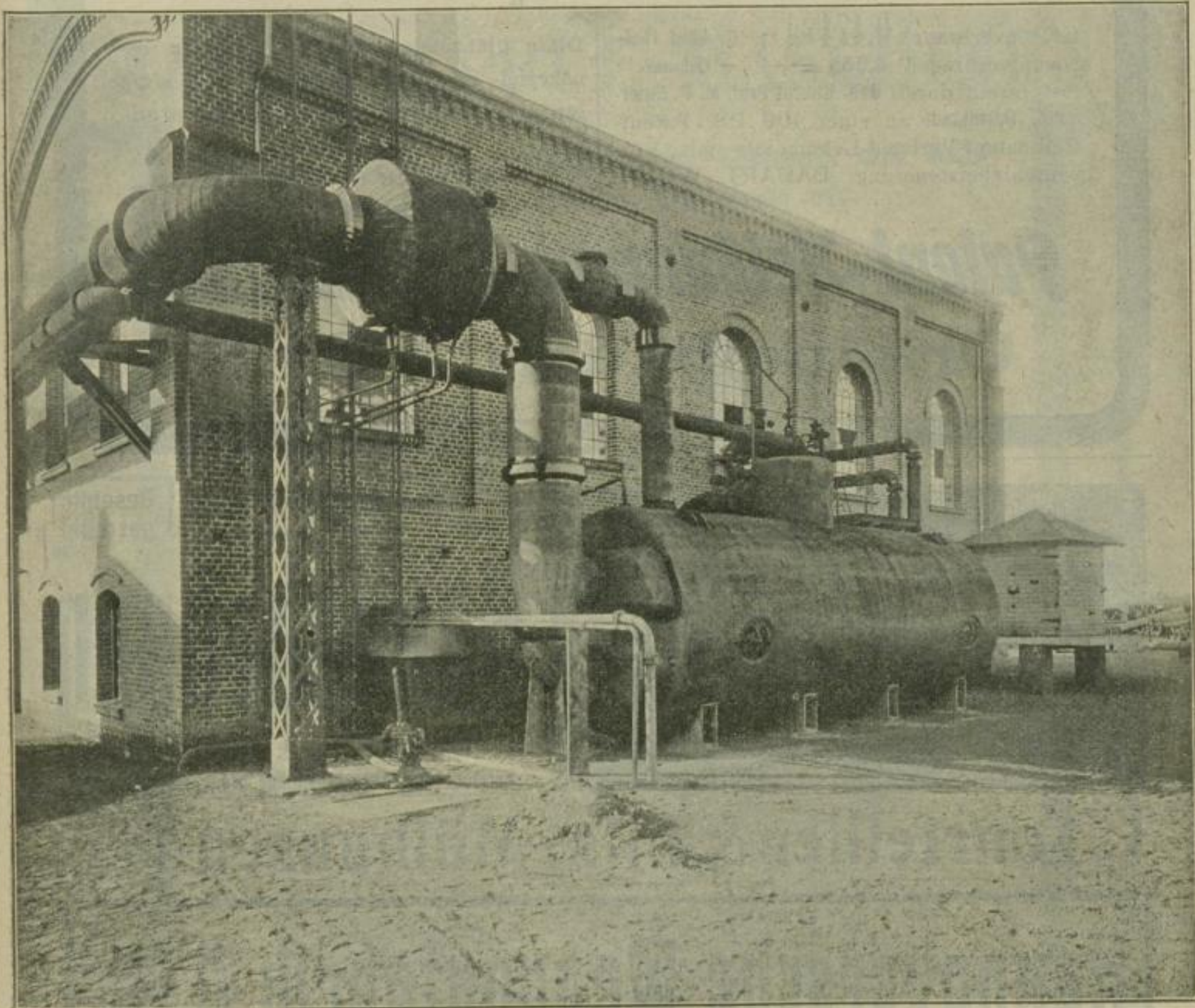
Wärmespeicheranlage zum Turbokompressor auf Zeche Concordia, Schacht 2, Oberhausen.
