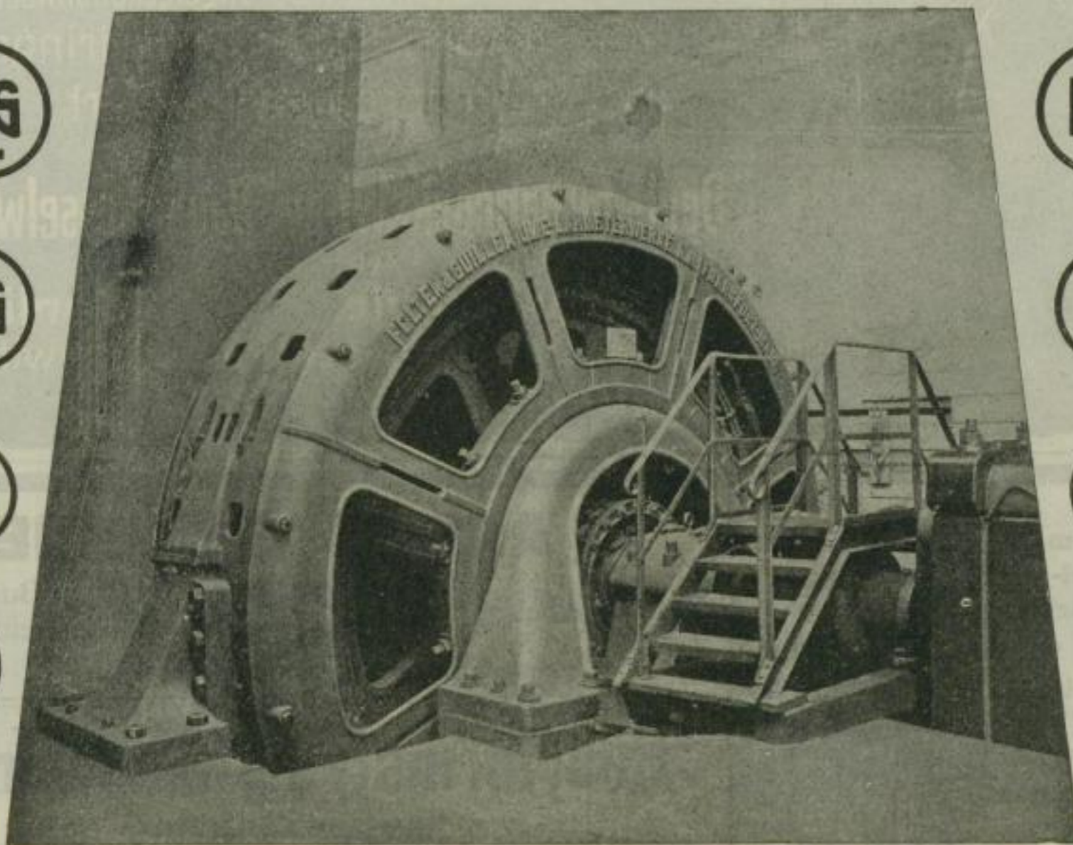
Drehstrommotor zum Antrieb einer Drahtstraße. Normalleistung 2000 PS., 100 Umdrehungen i. d. M., 150 % Überlastbarkeit.
