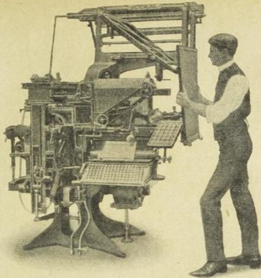
Viktorline (frühere Herkules) der General Composing Comp.; erbaut unter Benutzung abgelaufener Linotype-Patente
