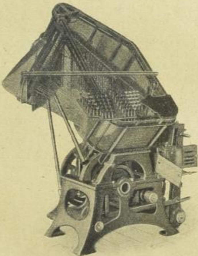
Linotype junior, erbaut von der amerikanischen Linotype-Gesellschaft, die bekanntlich die Typograph-Patente übernahm. Der Kreislauf der Linotype-Matrizen ist auch bei diesem Typographtyp durchgeführt
